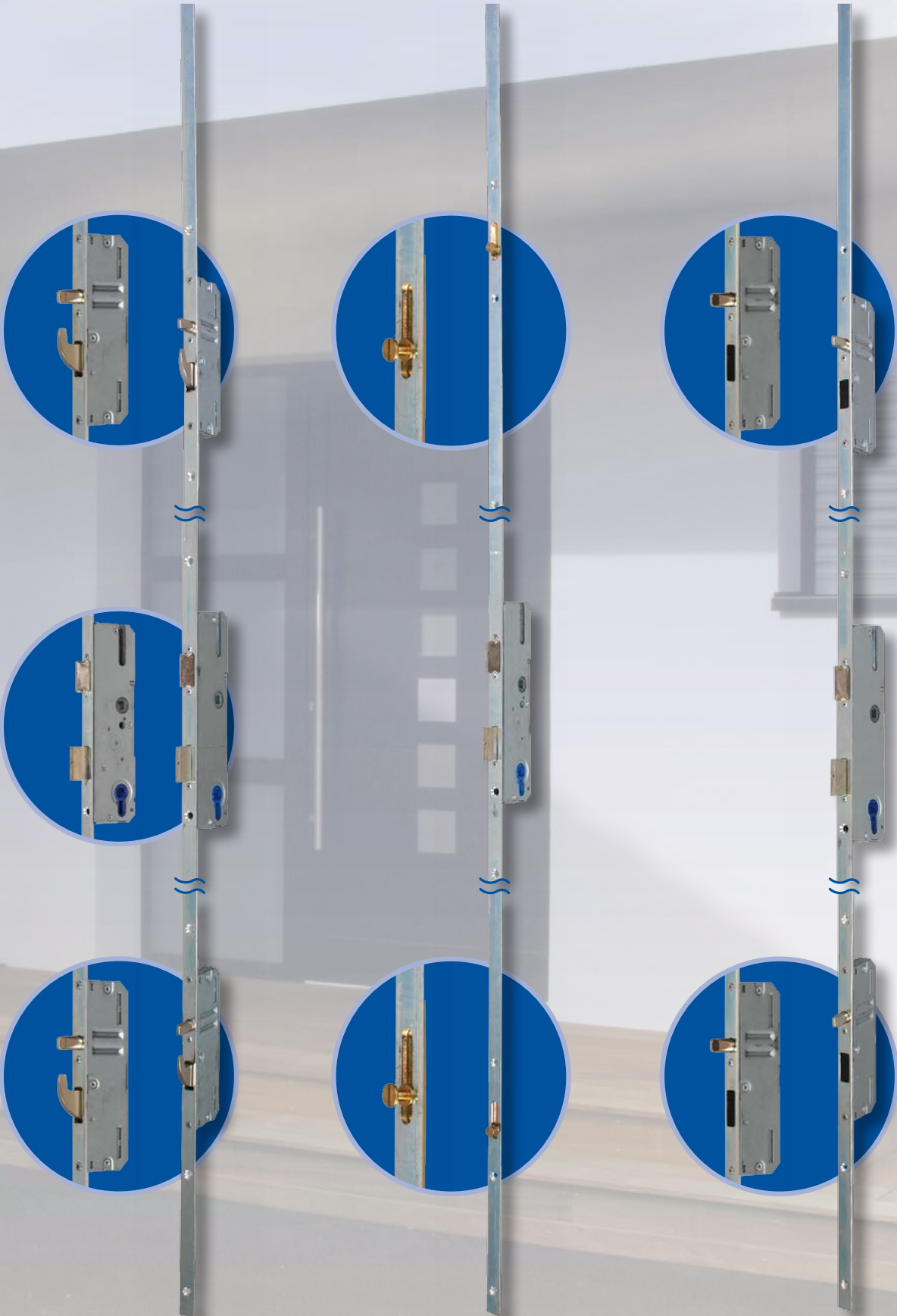
Serrure 5 points dont 2 crochets
